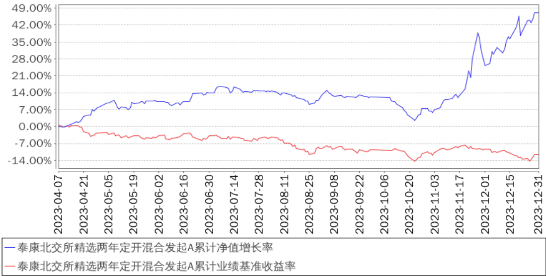
泰康北交所精选两年定开混合发起A累计净值增长率与同期业绩比较基准收益率的历史走势对比图
