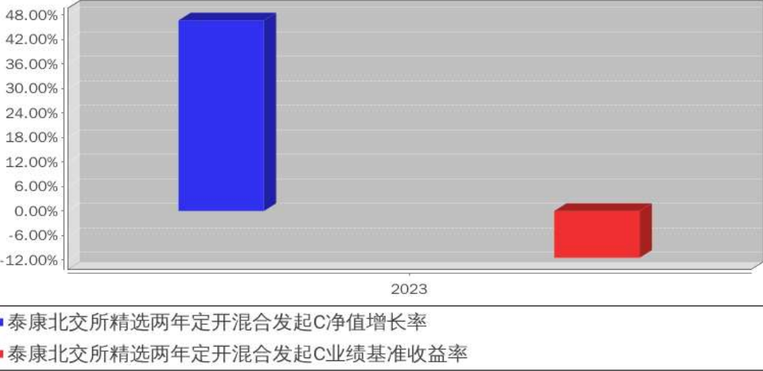
泰康北交所精选两年定开混合发起C基金每年净值增长率与同期业绩比较基准收益率的对比图
